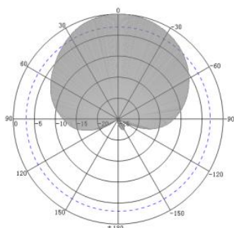
915MHz H-Plane
