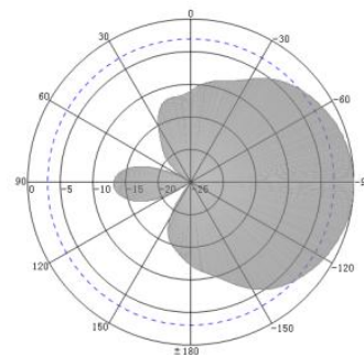
915MHz E-Plane
