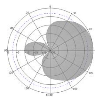
915MHz E-Plane
