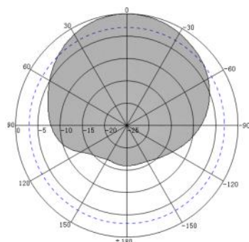
915MHz H-Plane
